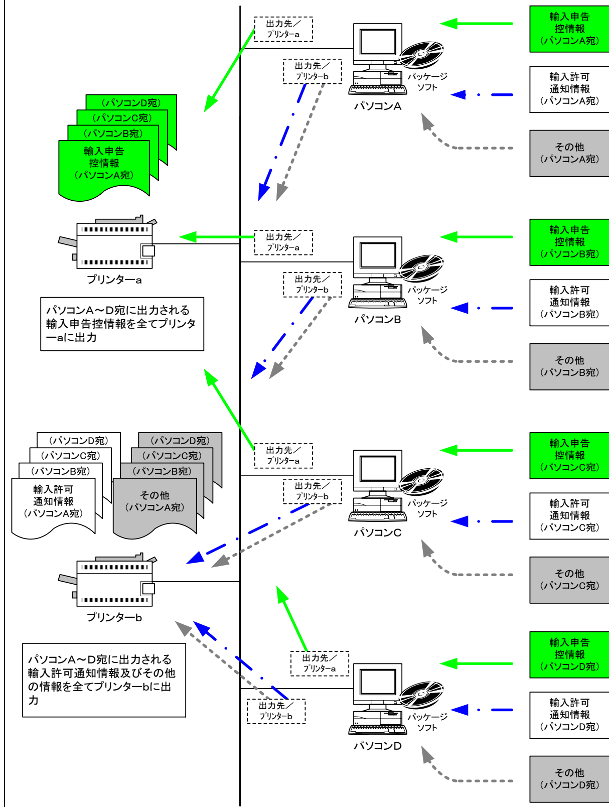
図 5-2-3 出力先プリンター設定のイメージ図②
