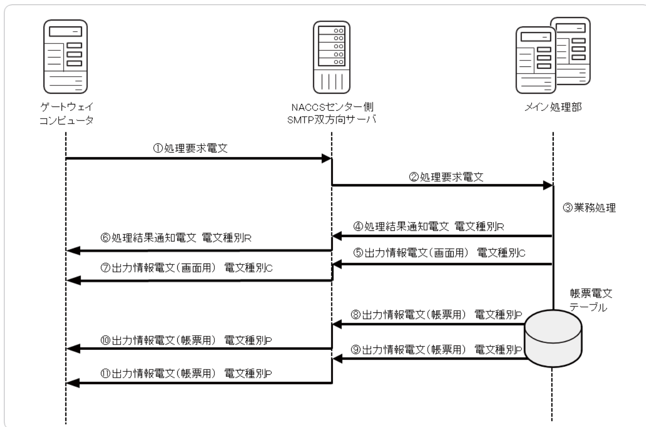
図 4-2-13 インタラクティブ処理方式（SMTP 双方向）の処理例
