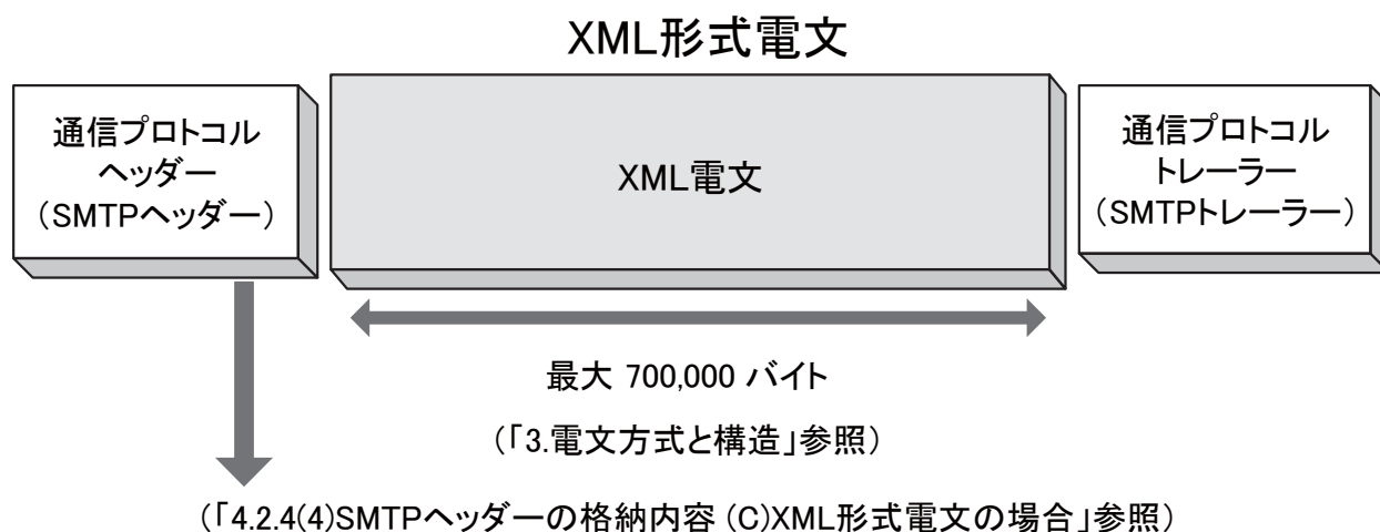
図 4-2-9 XML 形式電文の概要（インタラクティブ処理方式（SMTP 双方向））
