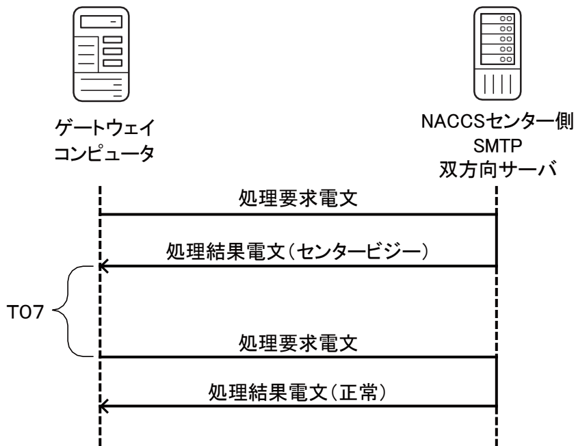
図 4-2-17 センタービジーの場合のタイマー設定
