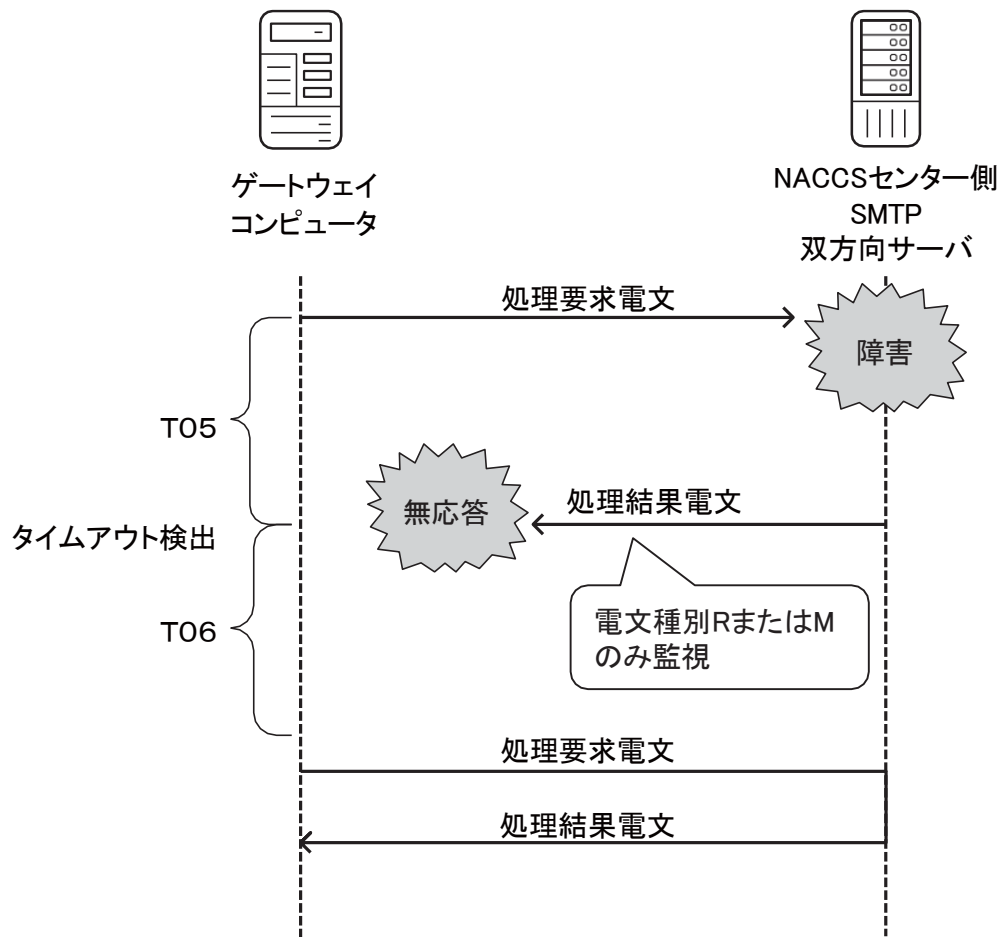
図 4-2-16 処理結果電文のタイマー監視
