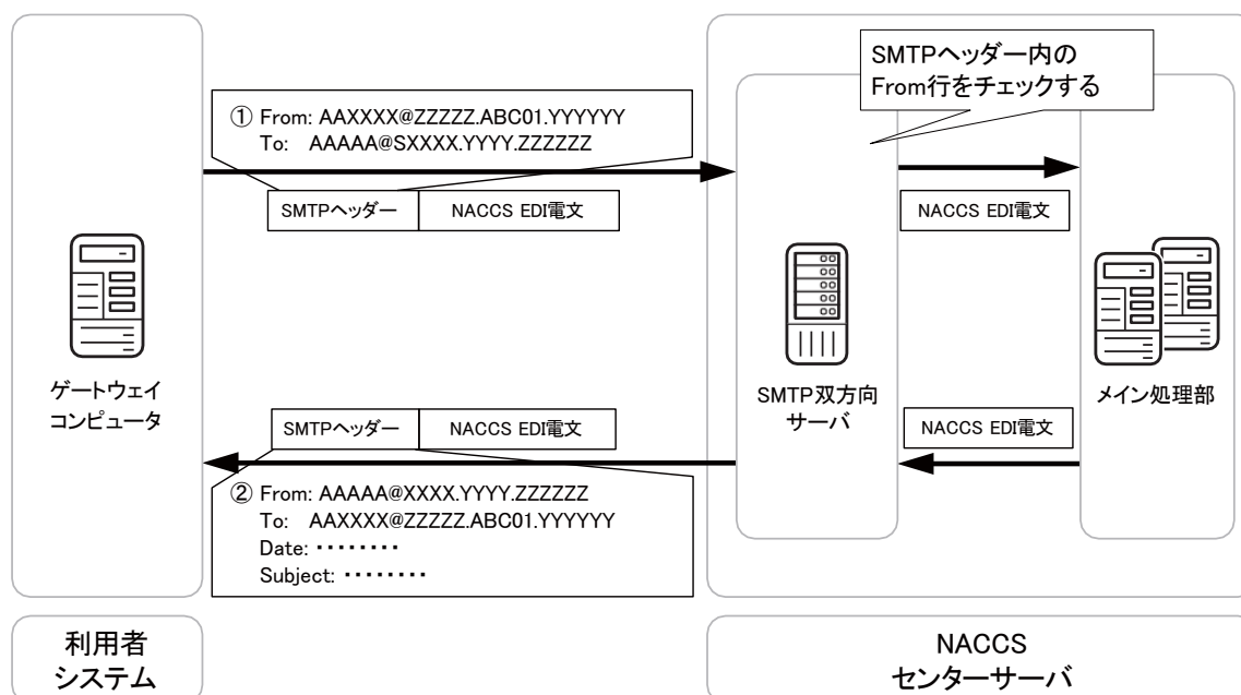
図 4-2-10 SMTP ヘッダー内のメールアドレス
