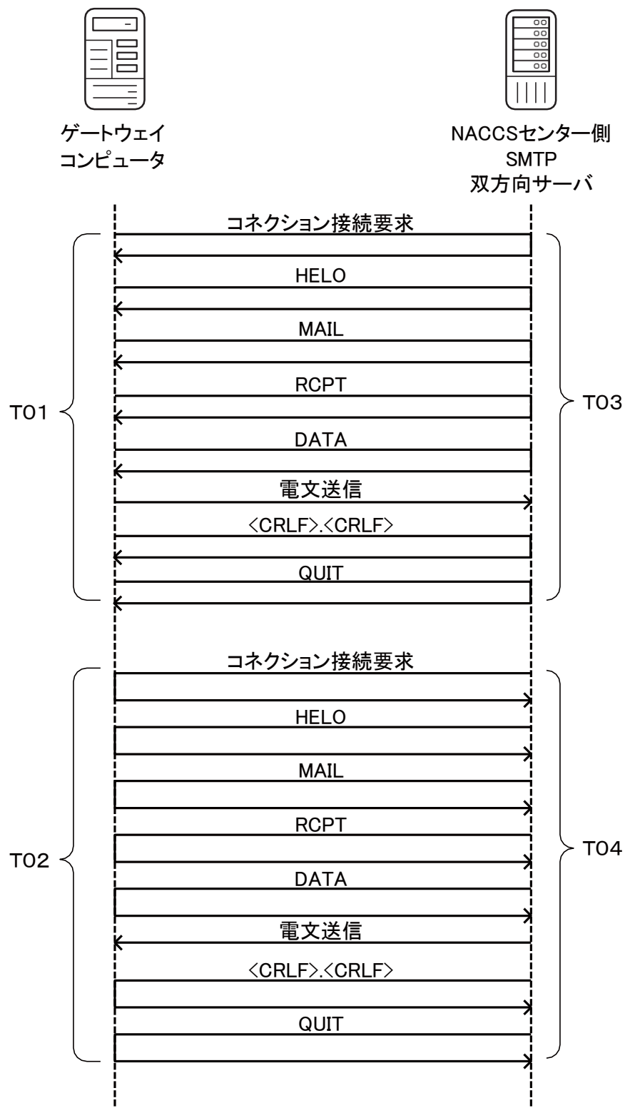
図 4-2-15 通常通信時のタイマー設定
