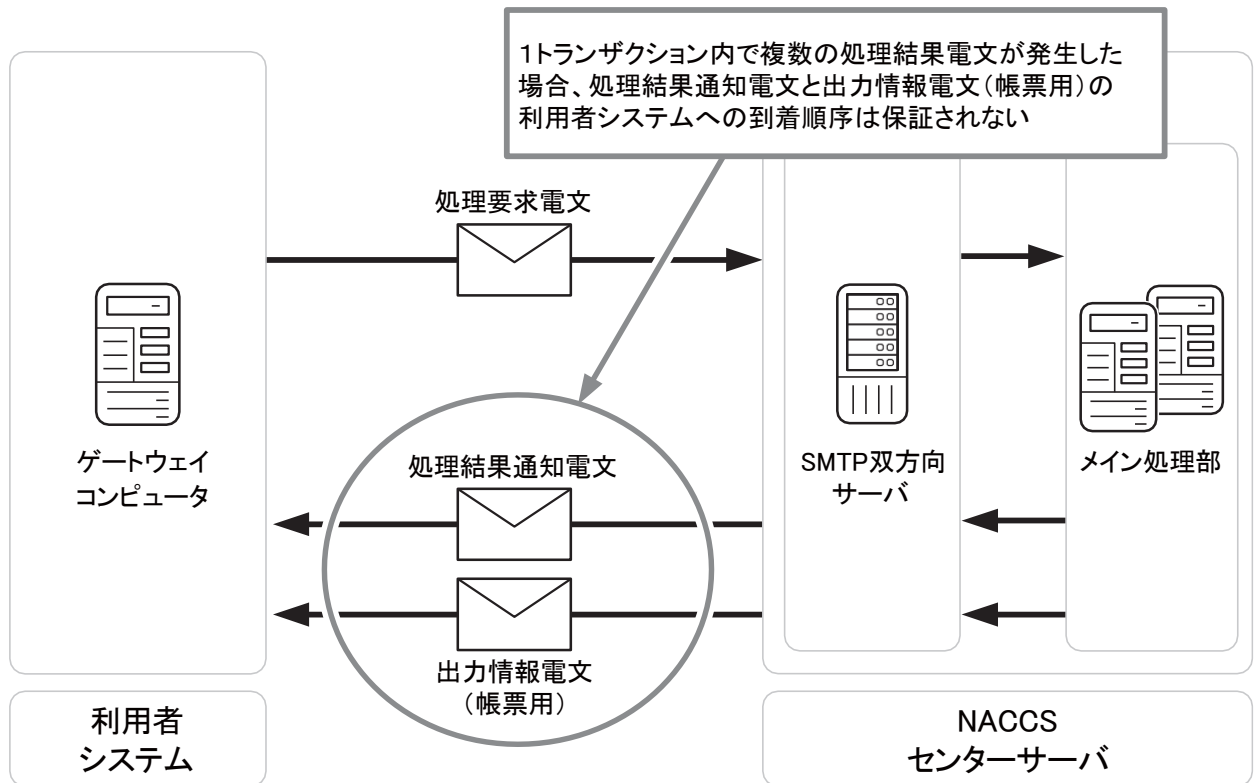
図 4-2-14 複数の処理結果電文の到着順序について (例)
