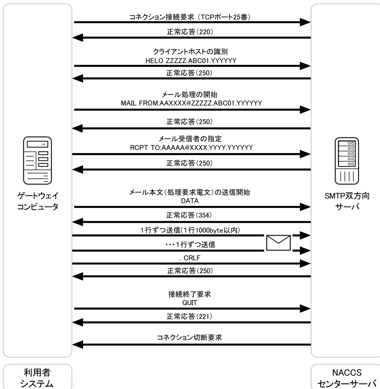
図 4-2-3 処理要求電文送信時の SMTP コマンドシーケンス
