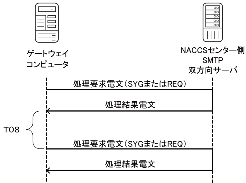
図 4-2-18 SYG 業務、REQ 業務のタイマー設定
