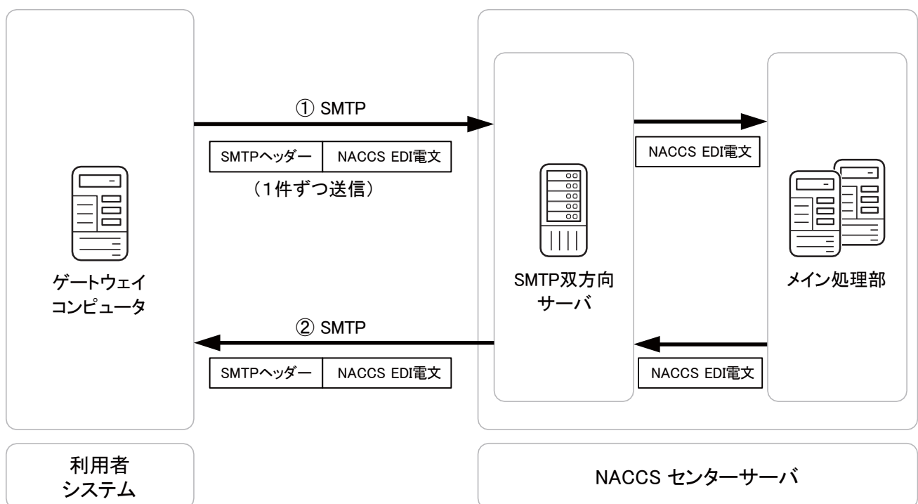
図 4-2-1 インタラクティブ処理方式（SMTP 双方向）の処理方式概要
