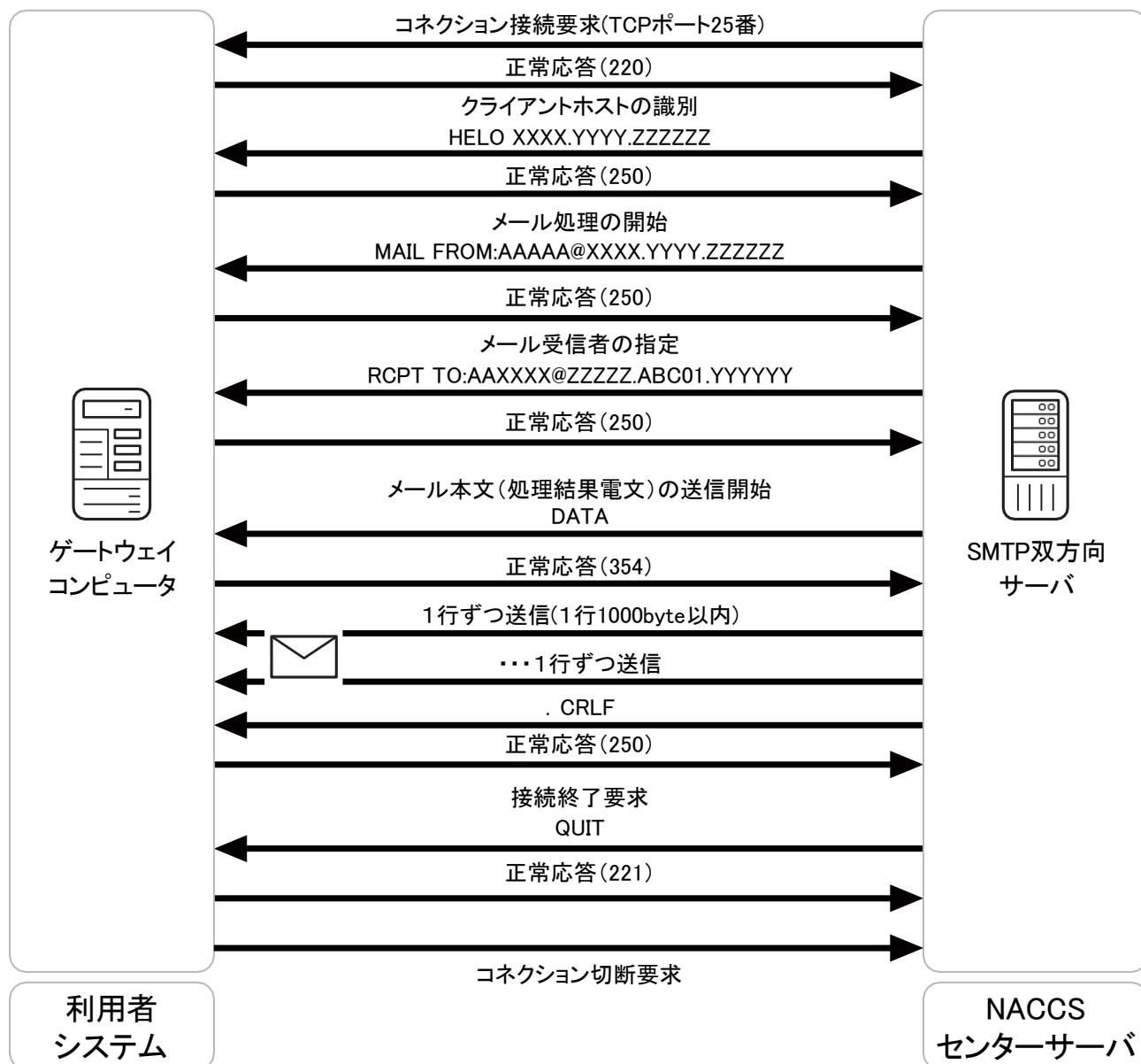
図 4-2-4 処理結果電文受信時の SMTP コマンドシーケンス
