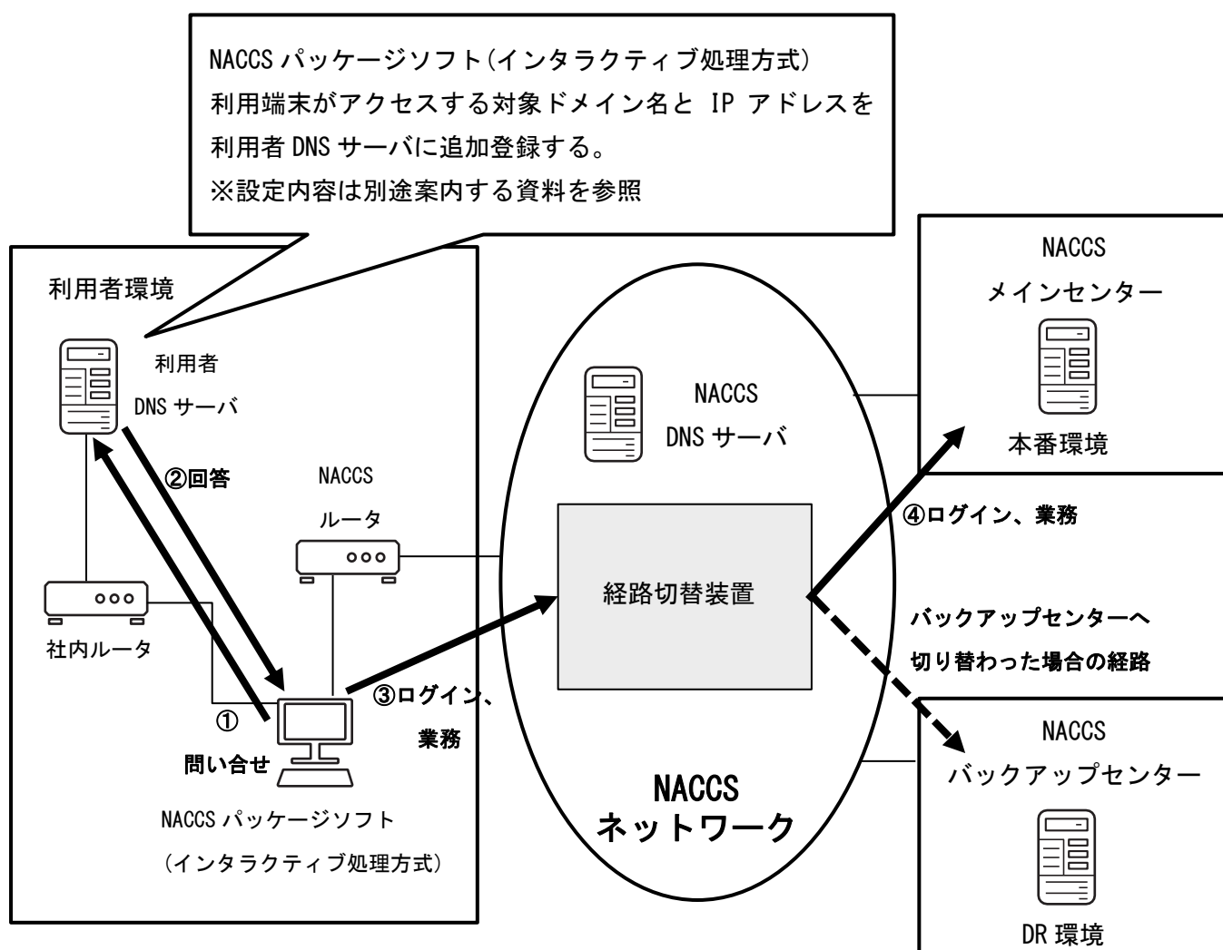
図 2-4-2 利用者環境と NACCS 全体の概要図
